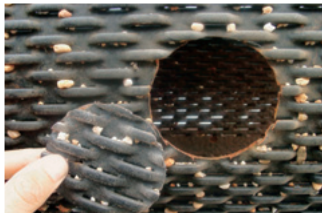
Abb. 4 Durch Unterkorn kolmatierter Schlitzbrückenfilter (aus aufgelassenem Brunnen)
