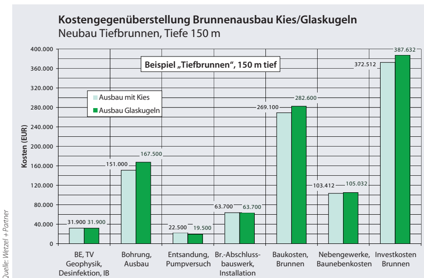
Abb. 6 Kostenanteile Teilgewerke „Tiefbrunnen“
